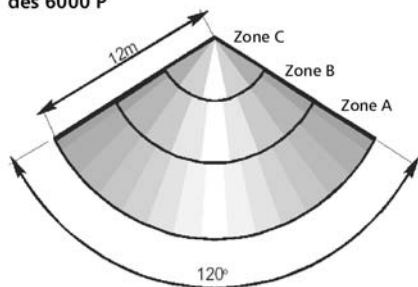
Erfassungsbereich des 6000 P
